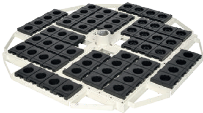
Exemple: Cadre équipé avec inserts d'outils E2
